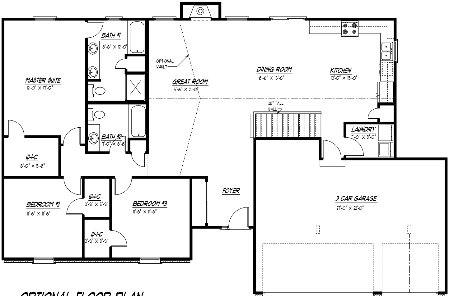
OPTIONAL FLOOR PLAN
